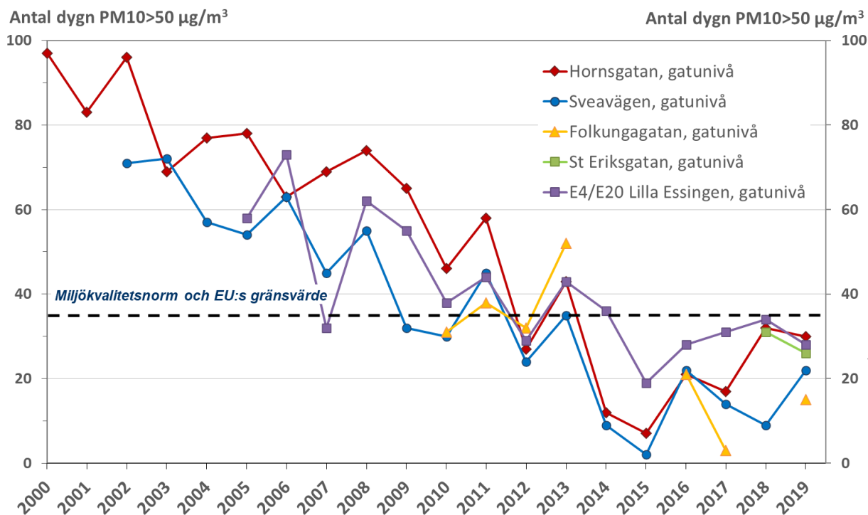
Figur 7. Trender för partiklar, PM10, antal dygnsmedelvärden högre än normvärdet 50 \mu\text{g}/\text{m}^3 under perioden 2000–2019.
