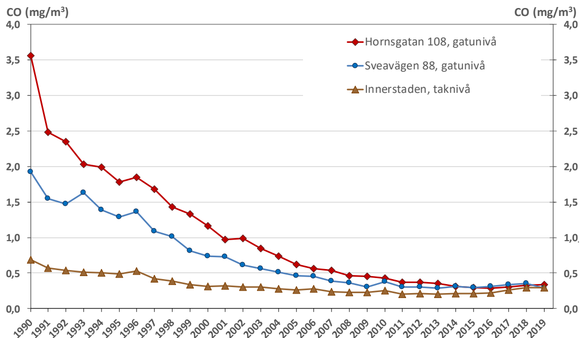
Figur 13. Trender för årsmedelvärden av CO under perioden 1990–2019 vid mätstationerna på Hornsgatan och Sveavägen. Halterna av CO i taknivå är ett medelvärde av Hornsgatan och Sveavägen.
