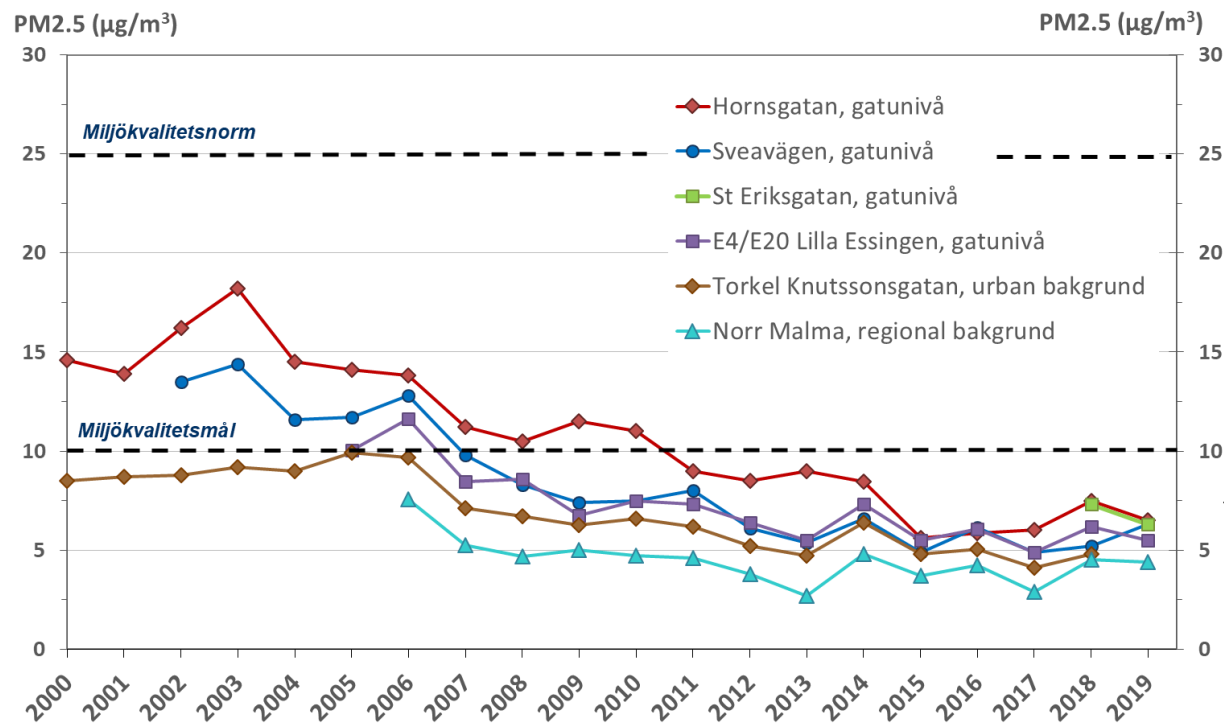
Figur 10. Trender för uppmätta årsmedelvärden av partiklar, PM 2.5 , för perioden 2000–2019.
