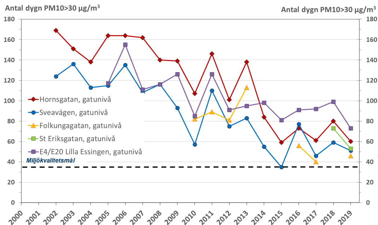
Figur 8. Trender för partiklar, PM10, antal dygnsmedelvärden högre än målvärdet 30 µg/m³ under perioden 2000–2019.
