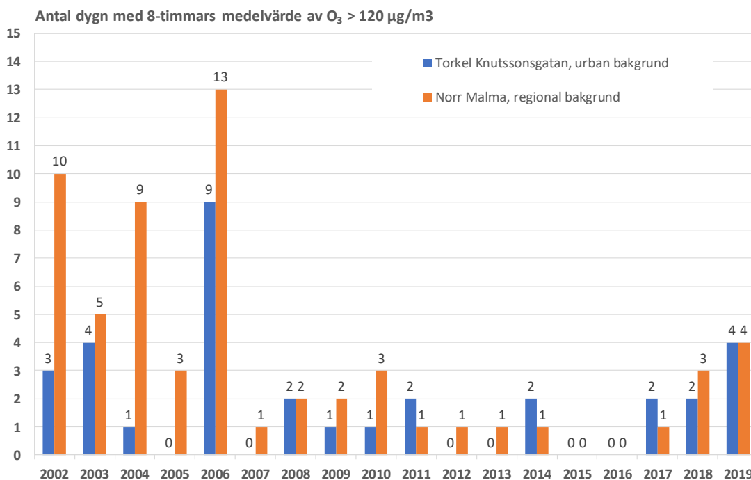
Figur 17. Trender för antal dygn med ozonhalter högre än normvärdet 120 \mu\text{g}/\text{m}^3 åren 2002–2019.
