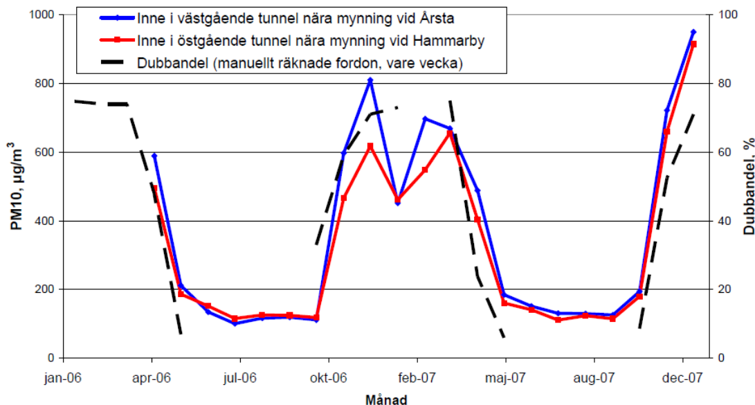
Figur 2. Månadsmedelvärden av PM10-halter i Södra länken tunneln
